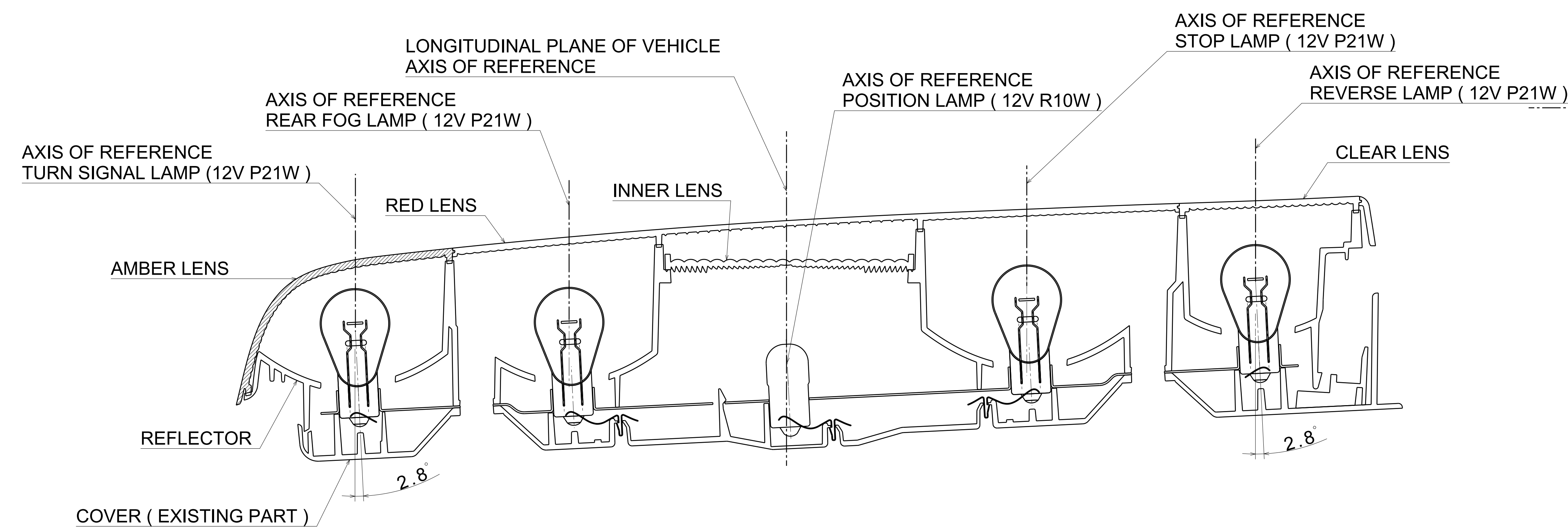
SECTION A-A
